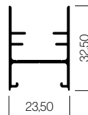
Profilo Fisso 27 042098
