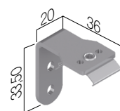
Soporte pared 029226
