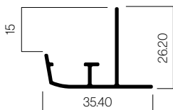
Avant guide 031241
