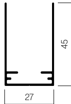
Upper guide 27 042099
