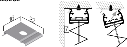
Soporte techo 029202
