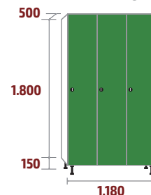
FV-40/3 COD: 53113 120,8kg · 1,06m 3
