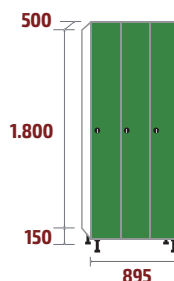
FV-30/3 COD: 53102 104,3kg · 0,81m 3
