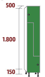
FL-40/1 COD: 53042 56kg · 0,36m 3
