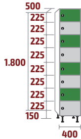
FZ-40/1 COD: 53082 70kg · 0,36m 3
