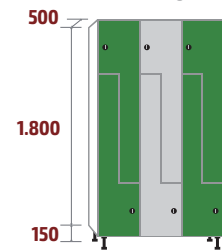
FL-40/3 COD: 53185 150kg · 1,06m 3
