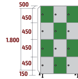
FC-40/3 COD: 53145 143kg · 1,06m 3
