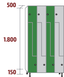
FL-30/4 COD: 53183 175kg · 1,07m 3
