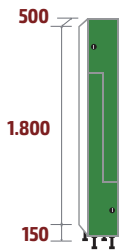
FL-30/1 COD: 53041 51kg · 0,27m 3
