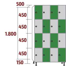
FC-30/4 COD: 53143 158kg · 1,07m 3
