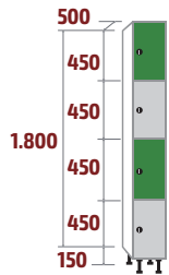
FC-30/1 COD: 53021 50kg · 0,27m 3
