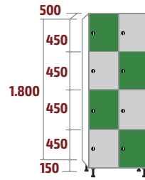
FC-40/2 COD: 53144 99kg · 0,71m 3
