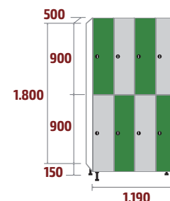
FT-30/4 COD: 53122 136,85kg · 1,07m 3
